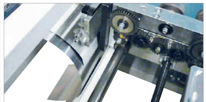
Coupe transversale partielle avec élimination de la chute
