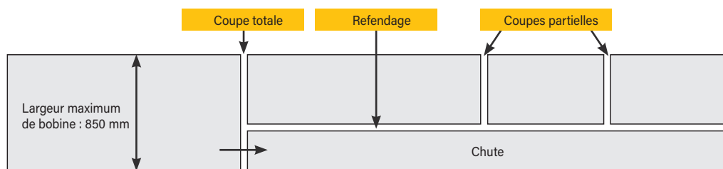
Coupe partielle avec élimination de la chute
