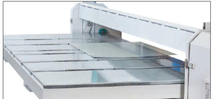
Butées arrières électriques, course maxi 750, 1000 ou 1500 mm - Réf. PTSL-BAE
